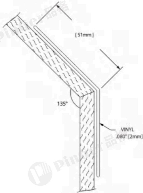
CG515结构图
